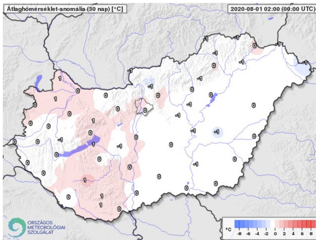
5. ábra: A hőmérsékleti anomália minimális volt júliusban
