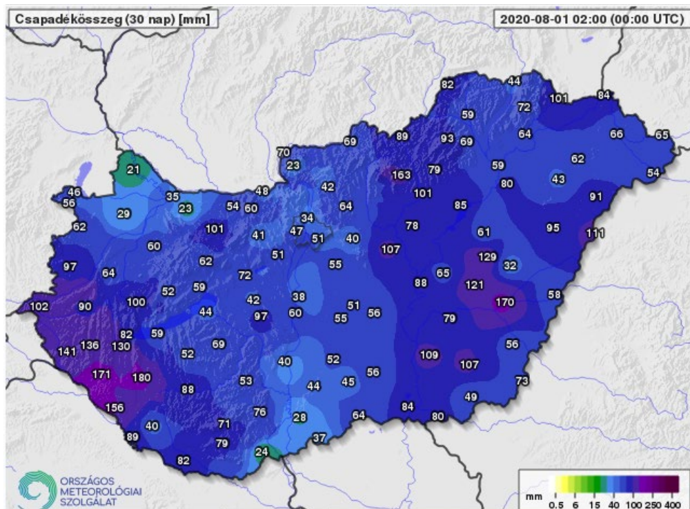
1. ábra: A júliusi (30 napos) csapadék eloszlása Magyarországon
