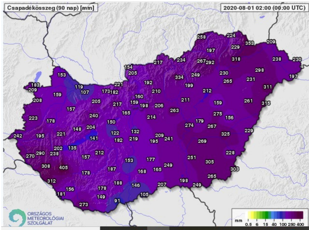
2. ábra: Háromhavi (90 napos) csapadékeloszlás Magyarországon
