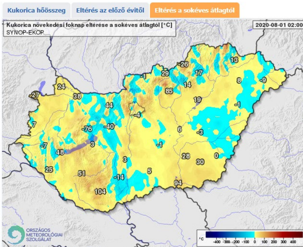
7. ábra: A növekedési foknap eltérései a sokéves átlagtól
