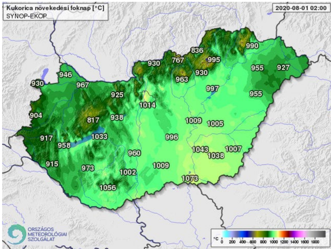
6. ábra: Magyarország hőegység térképe április 1-től augusztus 1-ig (Április 1-től a vetésidőig napi kb. 3 foknap vonható le)
